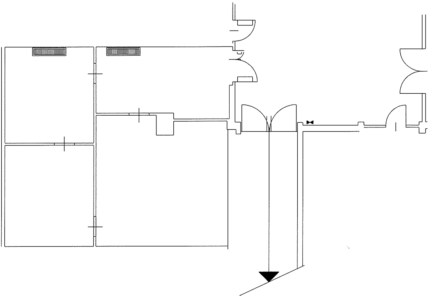
Piano seminterrato - zona A - mq. 100 circa - scala 1:100
