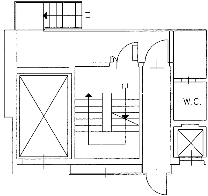
WC - Piano terra - zona A - scala 1:100
